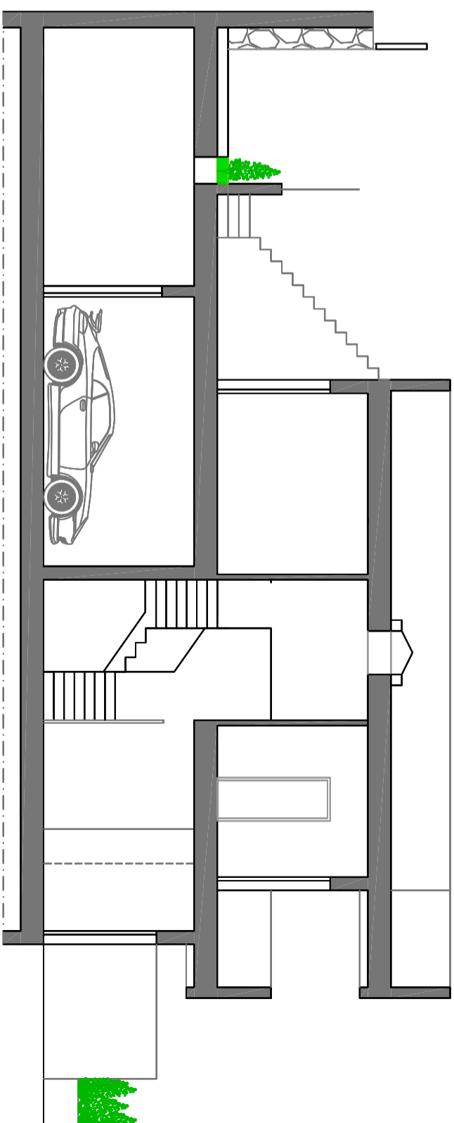
SECCIÓN LONGITUDINAL
