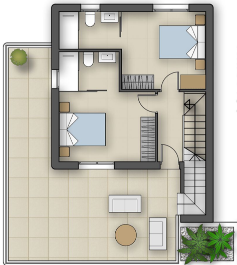
PLANTA PRIMERA / FIRST FLOOR
