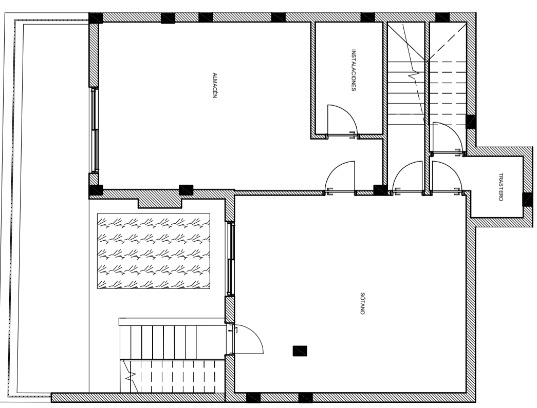
PLANTA SEMISÓTANO
