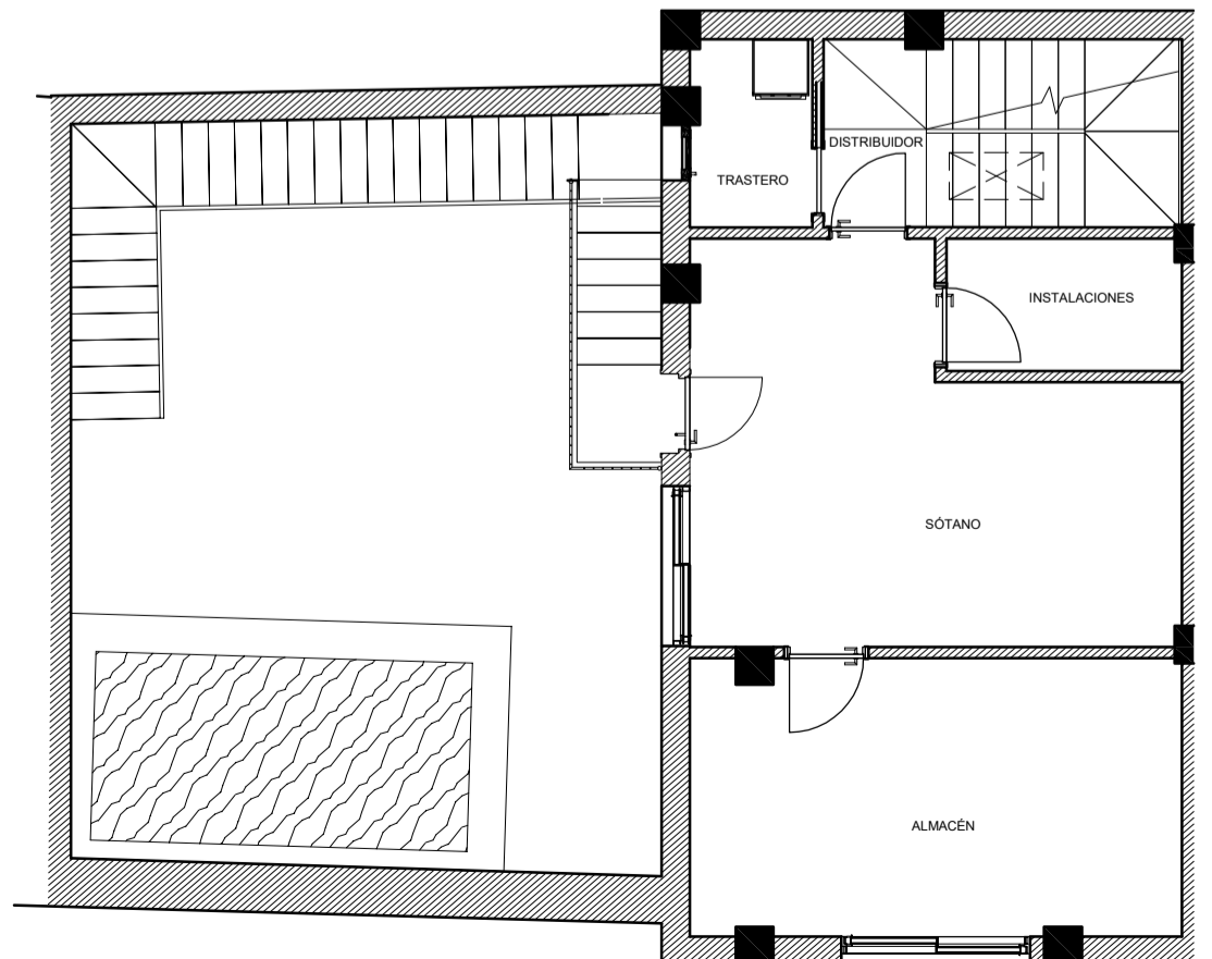
PLANTA SEMISÓTANO
