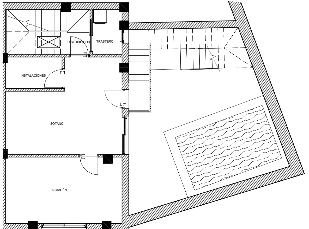
PLANTA SEMISÓTANO
