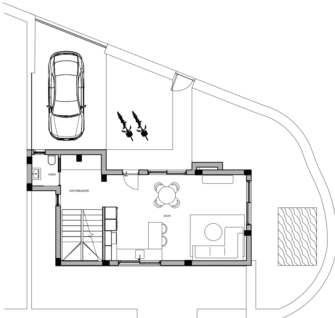
PLANTA -1 (NOCHE)
