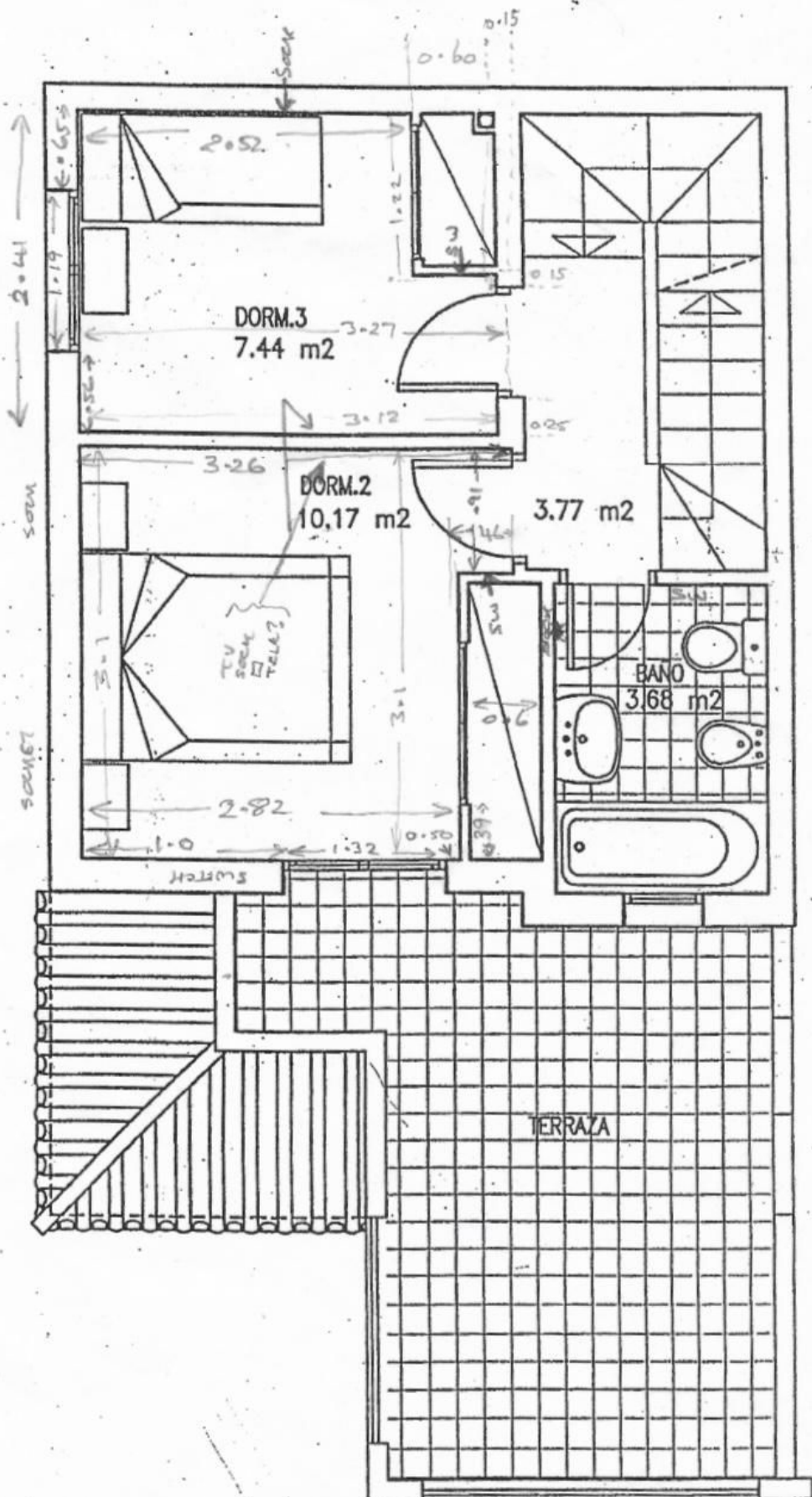
VIVIENDA DE 3 DORMITORIOS PLANTA PISO
