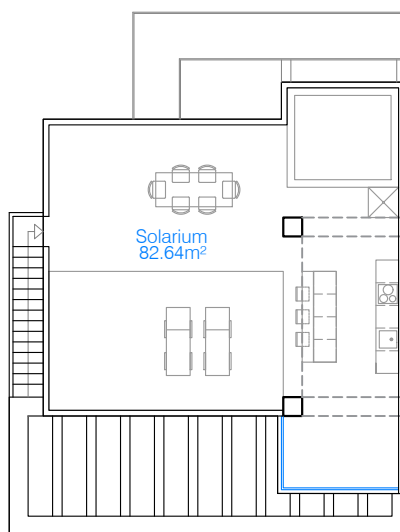
Solarium (E:1/200)
